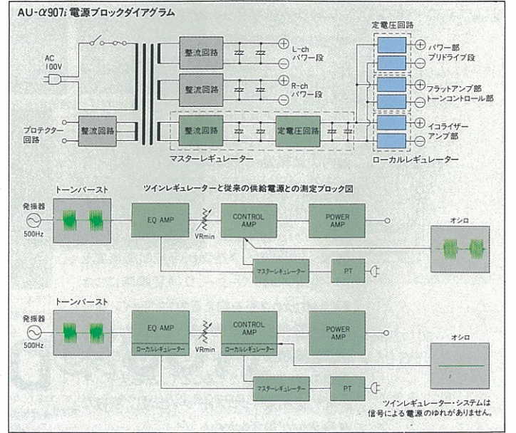
ツインレギュレーターシステムは、信号による電源のゆれがありません。
