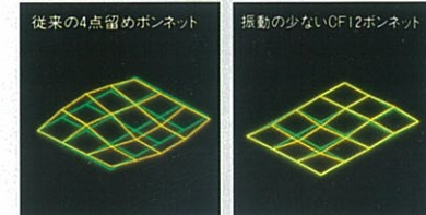
●ボンネットのモーダル解析比較。
