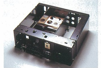
シールド特性を向上させた無振動、無共振設計の高剛性ソリッド&アンチフラックス・シャーシ。
